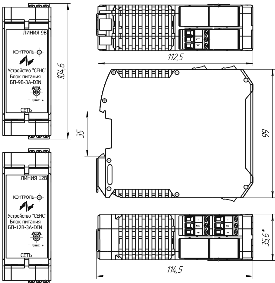
Рисунок Б.1. Внешний вид блоков питания, габаритные размеры, маркировка контактов.
